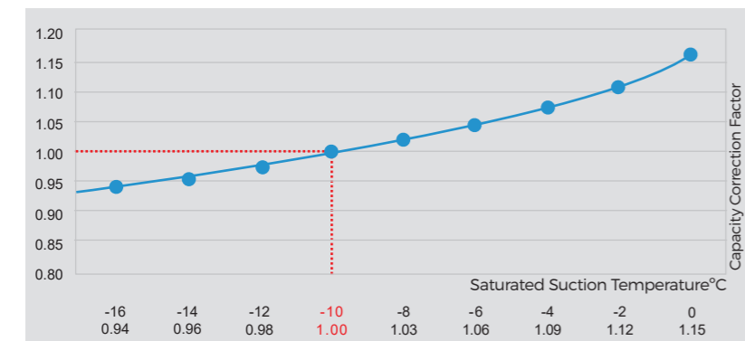
FLT...P Capacity Correction Graph
