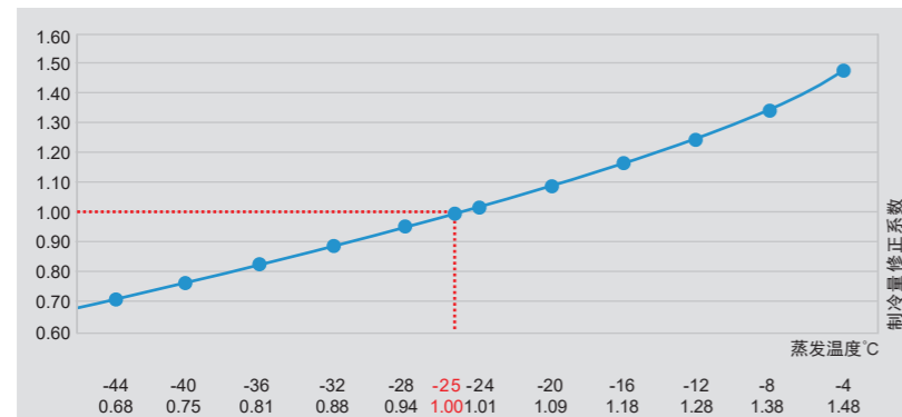
FLT 蒸发温度修正系数表
